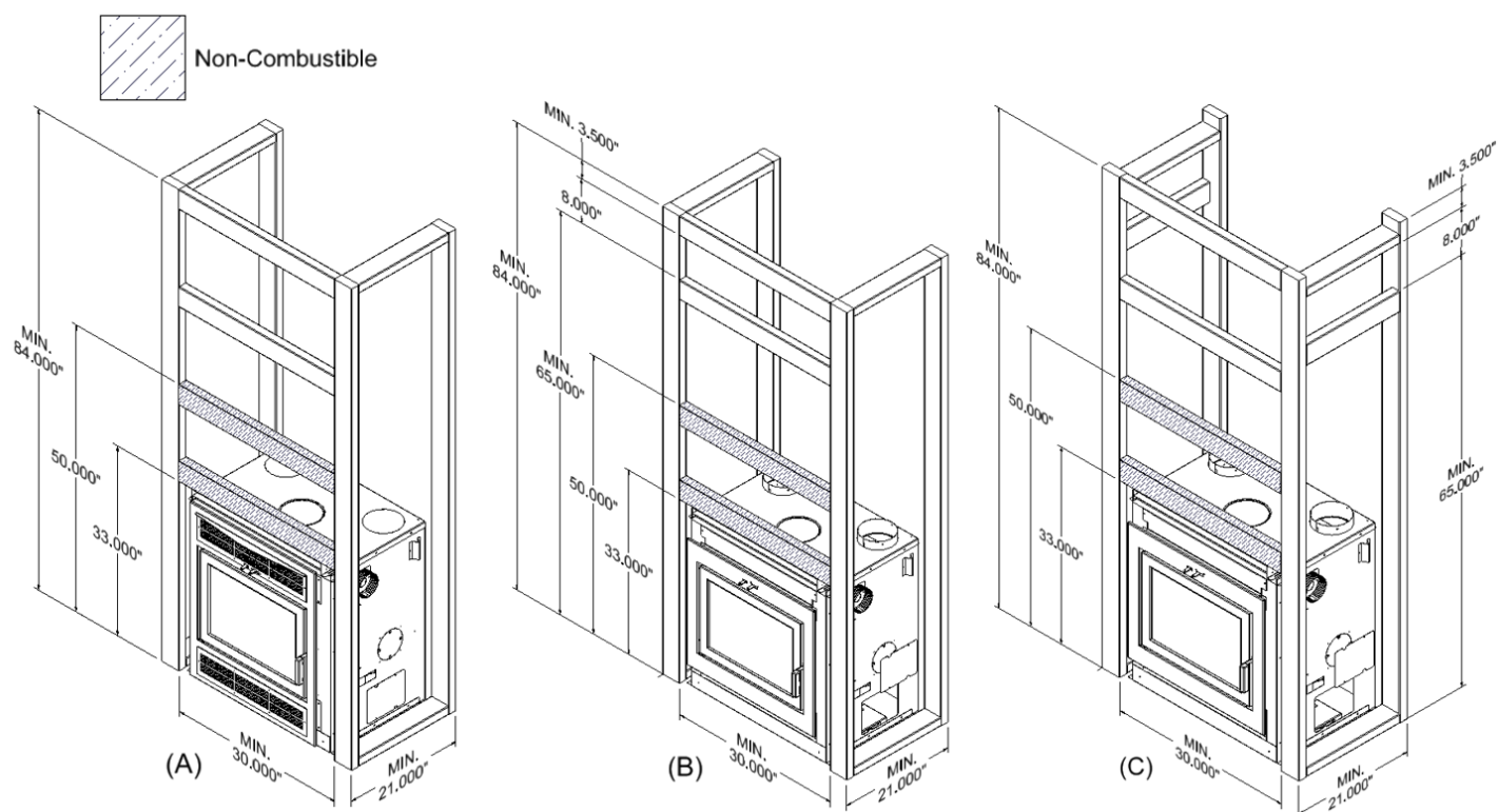
Figure 3-11: Charpente d'Élégance 30 pour (A) façade traditionnelle, (B) façade contemporaine avec sortie d'air chaud par gravité frontale et (C) façade contemporaine avec sortie d'air chaud par gravité latérale.
