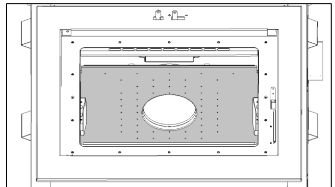
Illustration 2-3: Déflecteur de combustion secondaire à haute performance
