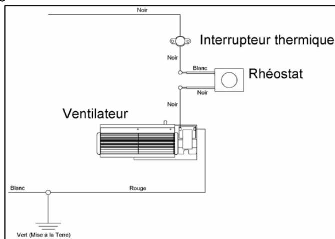
Illustration 3-21: Schéma électrique – Éléance 30
