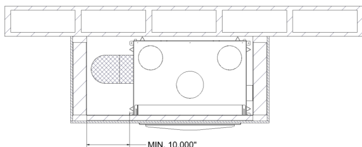
Illustration 3-1: Espace requis pour installer la prise d'air extérieur Voir section 4.1
