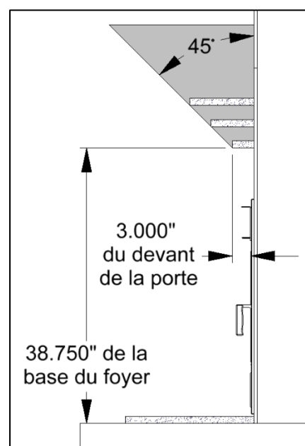
Illustration 3-18: Dégagement d'un manteau combustible
