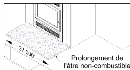
Illustration 3-13: Prolongement de l'âtre Élégance – Vue isométrique
