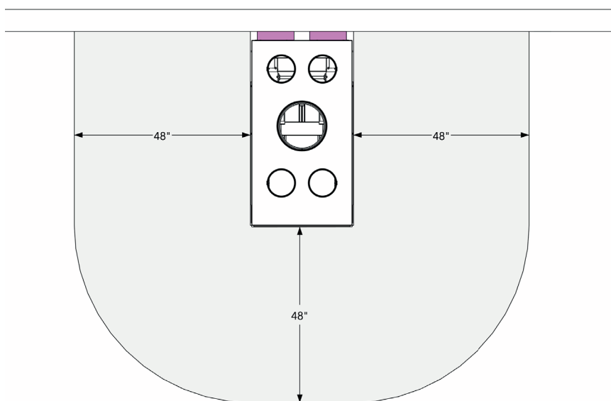
Foyers de type péninsule Dégagement minimale aux matériaux combustibles Exemple Luxus® Pier 28
