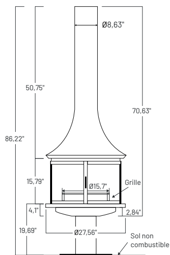
Vue de face (Centrale)
