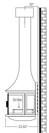
Vue de côté (Murale)
