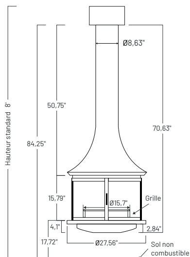
Vue de face (Centrale)
