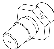
C Injecteur 1.3 Brûleur vertical - Droit
