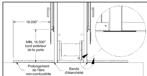
Illustration 3-12: Prolongement de l'âtre Éléance ST - Vue de côté
