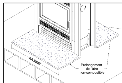
Illustration 3-11: Prolongement de l'âtre Éléance ST - Vue isométrique
