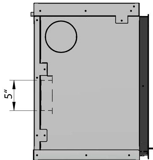
Entrée d'air à l'arrière du foyer
