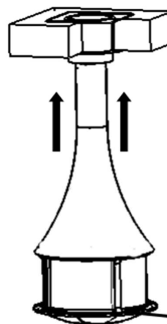
Fixation de la ZELIA908 - 3 vis TF M8x20
