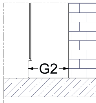
Illustration 3-12: Mesures de l'espace entre la maçonnerie et la façade du Flair
