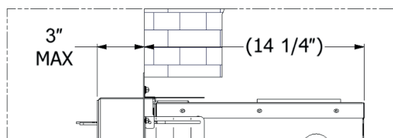
Illustration 3-15: FLAIR 25 Positionnement maximum de la moulure de finition
