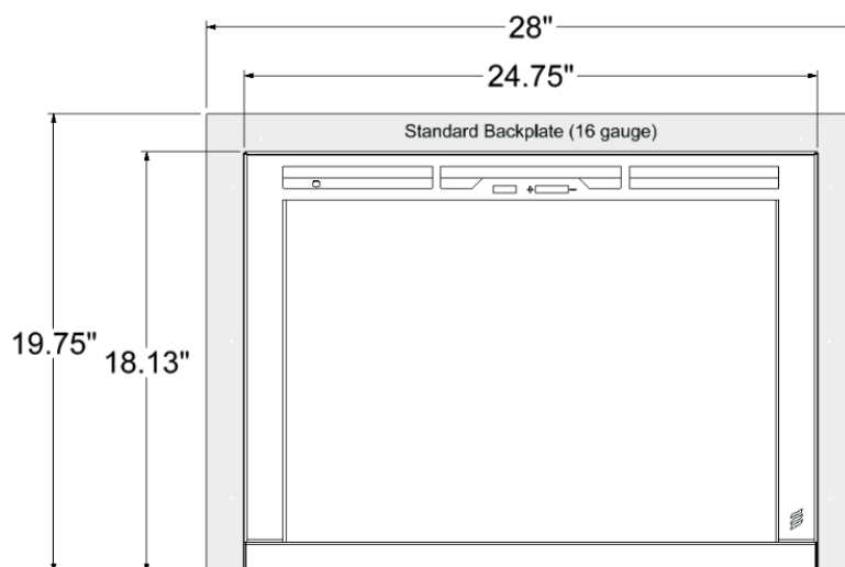
Illustration 2-7 : UWB200 - Façade FLAIR® 25
