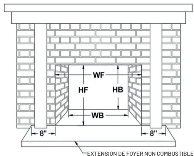
Illustration 3-2 : Dimensions ouverture minimal - Devant
