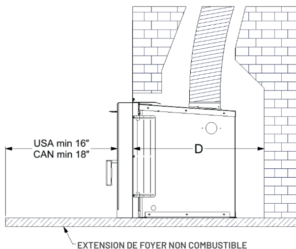
Illustration 3-1 : Dimensions ouverture minimal - Vue de côté
