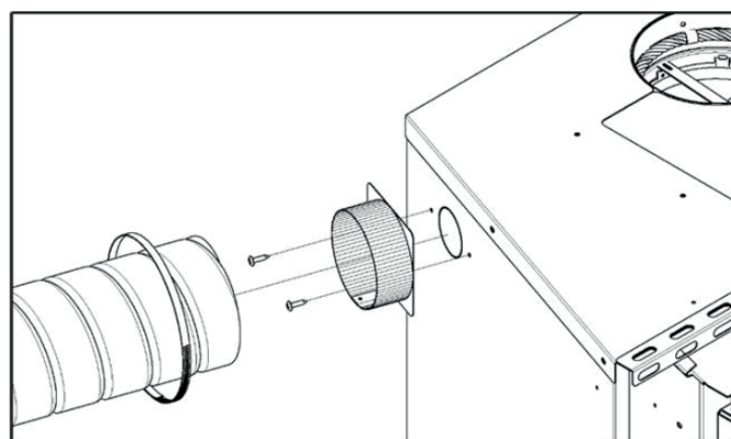
Illustration 4-5: Installation de l'ensemble d'air frais
