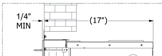
Illustration 3-13: FLAIR 25 Positionnement minimum de la moulure de finition
