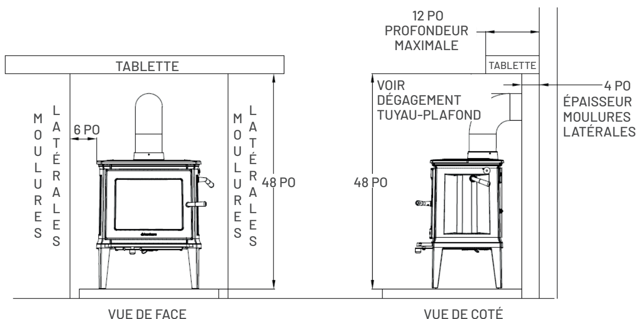
Figure 6 – Dégagements à la tablette et au manteau de foyer (combustible)
