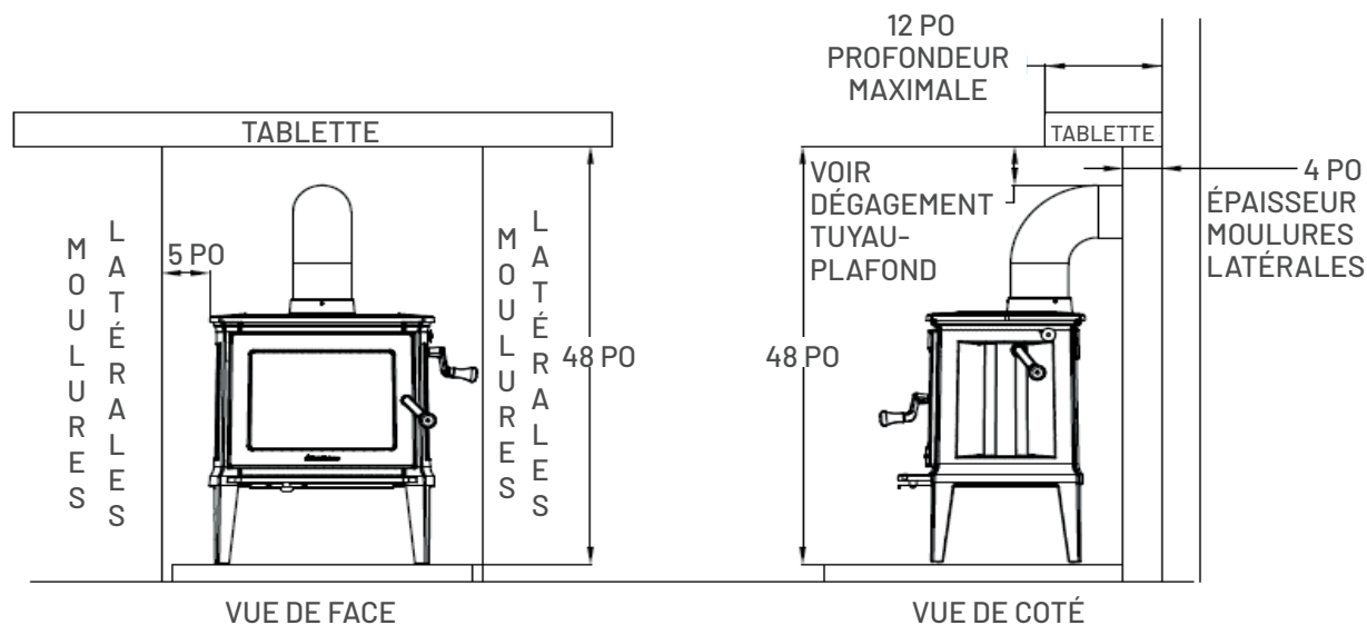
Figure 6 – Dégagements à la tablette et au manteau de foyer (combustible)
